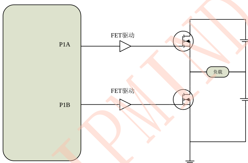
图 9.9a 标准半桥电路（推挽）
