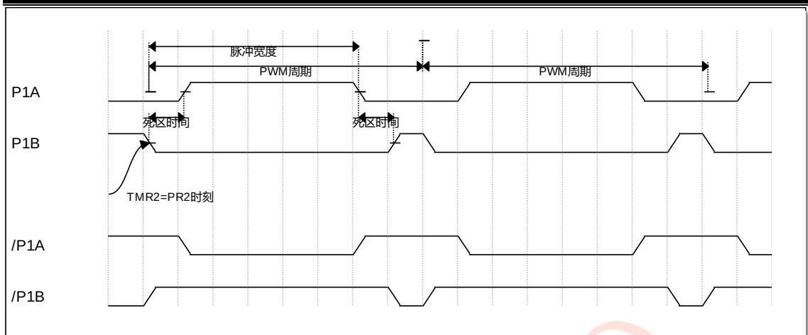
图 9.9d 半桥 PWM 输出（需要外接反相器）
