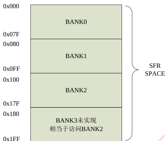
图 2.1.2 间接寻址
