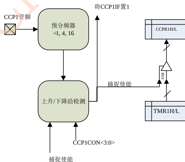
图 9.1 捕捉模式原理框图
