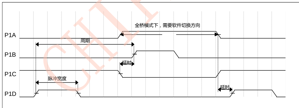
图 9.11b 全桥 PWM 输出示例 b
