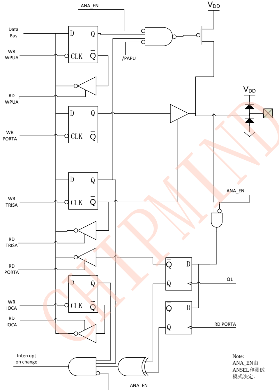
图 16.3 PA3 架构框图
