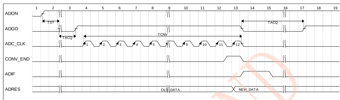
图 12.5 ADC 转换时序图
