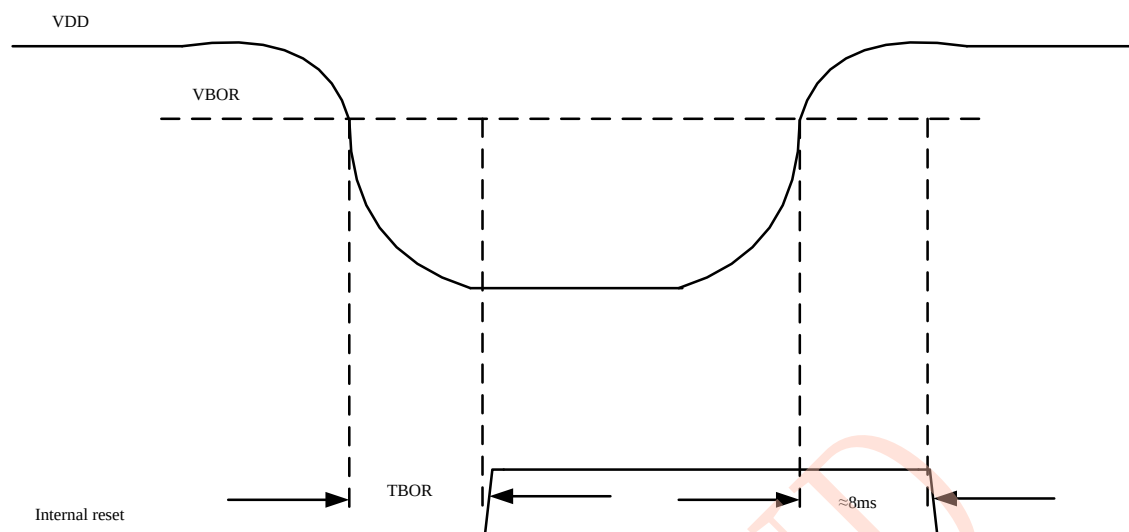
图 4.5 BOR 复位
